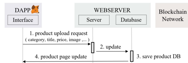
그림 7. 상품정보 업로드/갱신 절차
