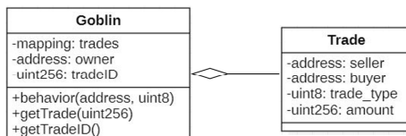
그림 12. 거래 기록 저장을 위한 구조체 구조
