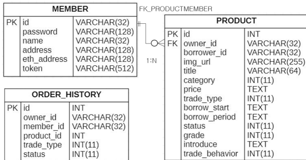
그림 5. 제안하는 공유 마켓 서비스를 위한 데이터베이스
