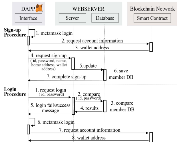
그림 6. 회원가입 및 로그인 절차
