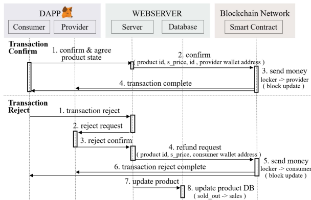
그림 9. 구매확정 및 환불 절차
