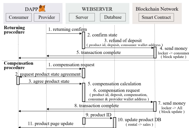
그림 11. 반납 및 배상 절차
